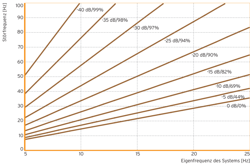
Abb. 4: Verminderung der Übertragung mechanischer Schwingungen durch den Einbau einer elastischen Lagerung aus Sylomer® SR 110 auf starrem Untergrund
